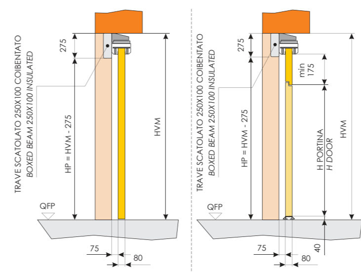
SENZA PORTINA PEDONALE WITHOUT PEDESTRIAN DOOR CON PORTINA PEDONALE WITH PEDESTRIAN DOOR
